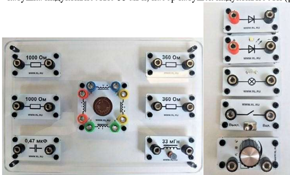
Рис. 7. Дополнительные элементы электрических цепей
